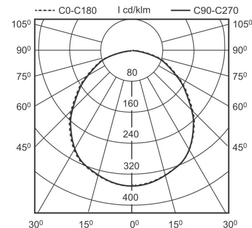
Рис. 2. Кривая силы света
